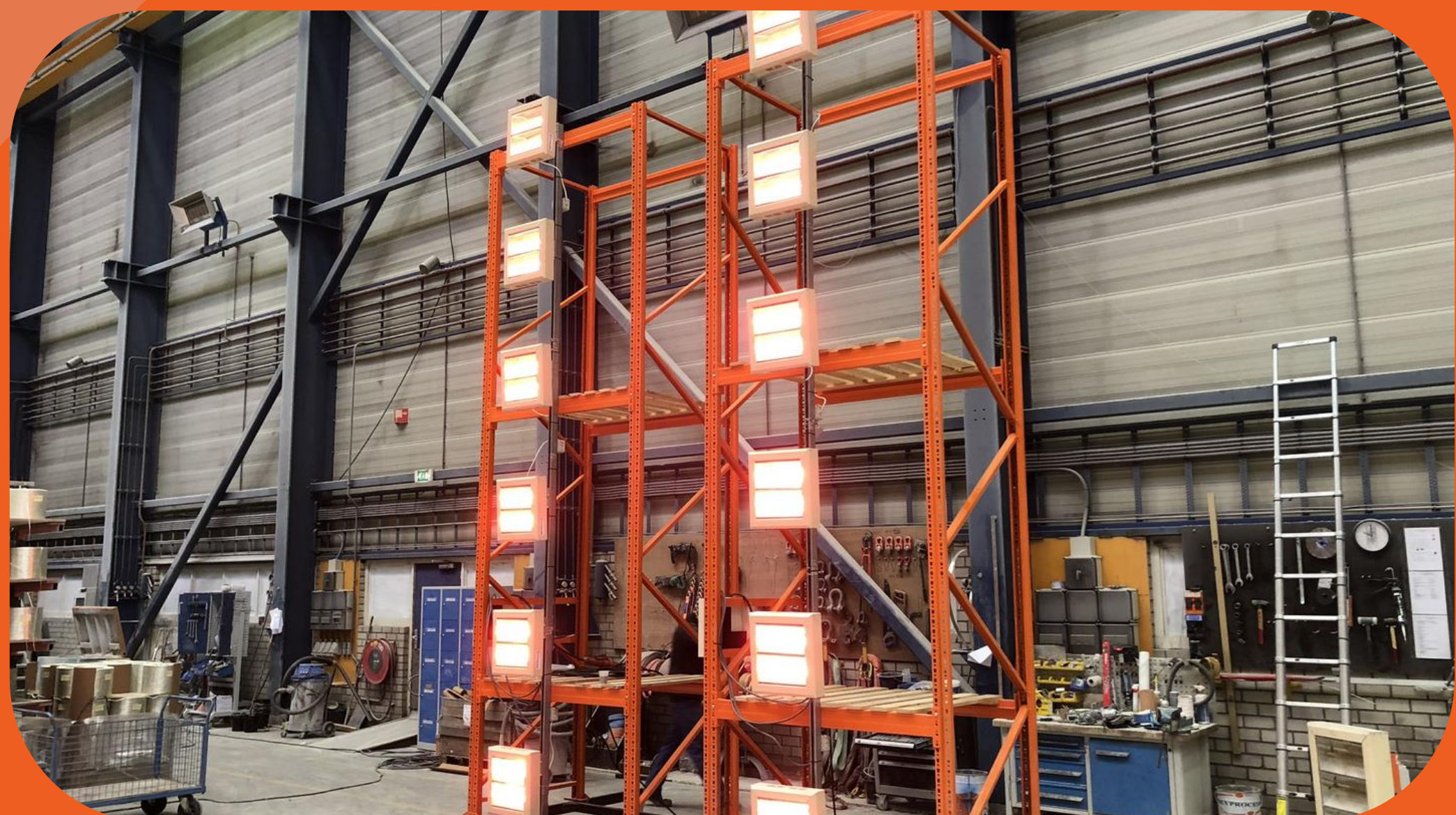
M.I.P. tanks & silo's - Rijkevorsel (België) Elektrische korte golf stralers
